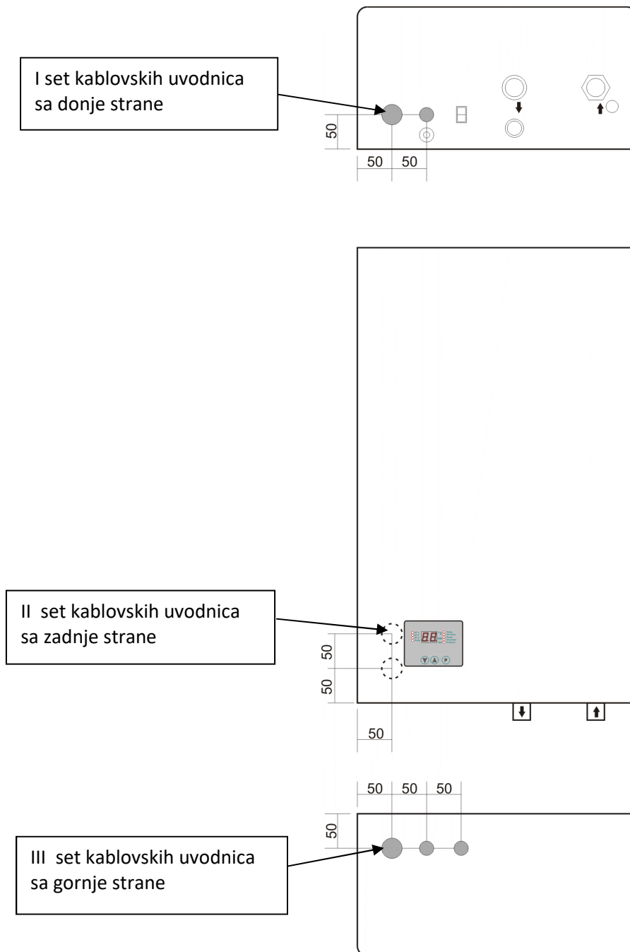
Slika: Prikaz pozicija uvodnica kablova na kotlu
