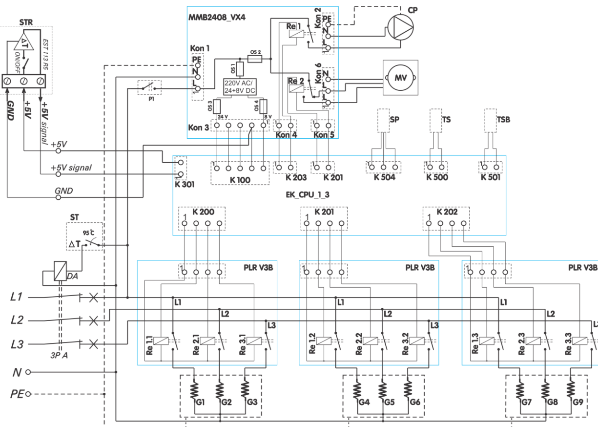
Figure 8: Schéma de commande de l'eTronic 7000
