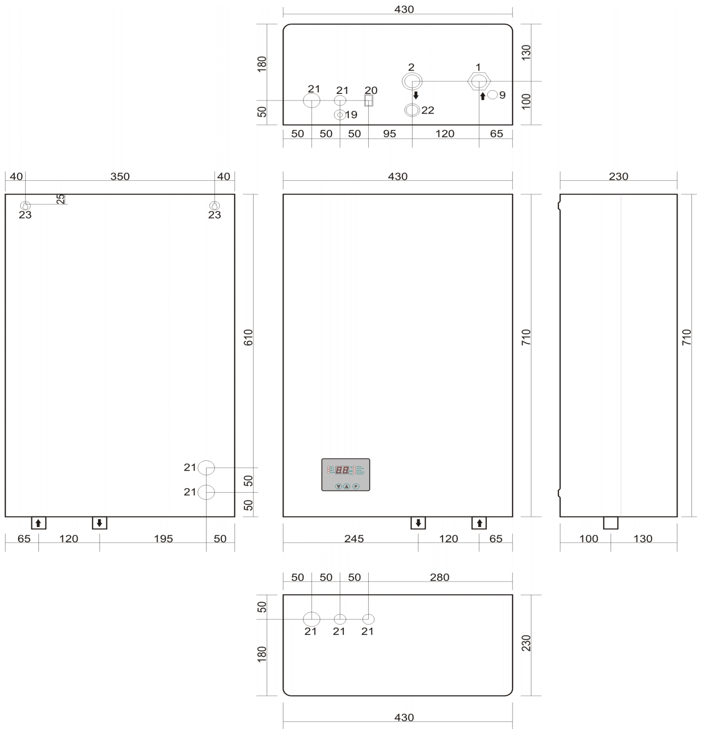
Slika: Dimenzije i priključci
