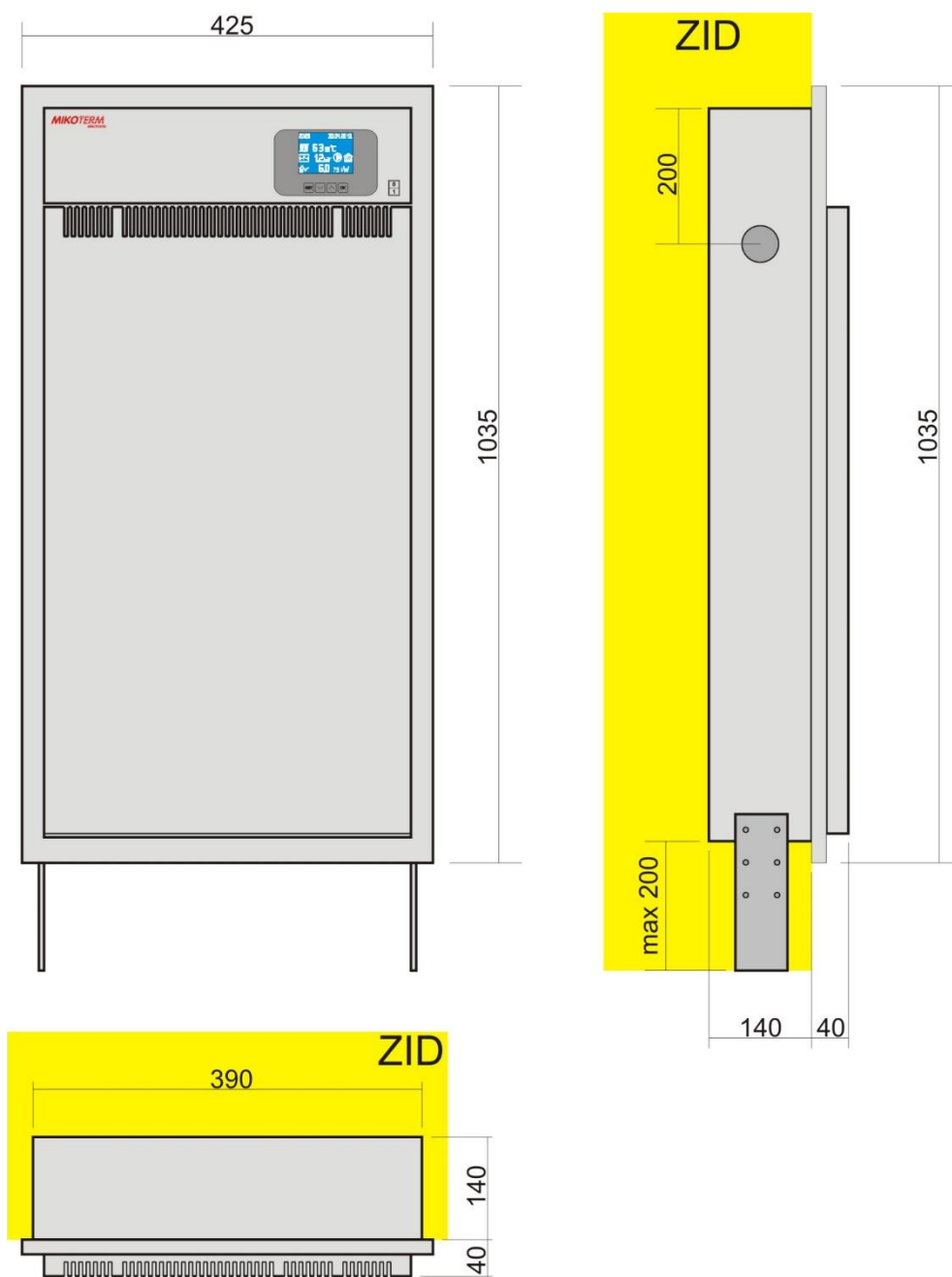
Slika: Dimenzije kotla
