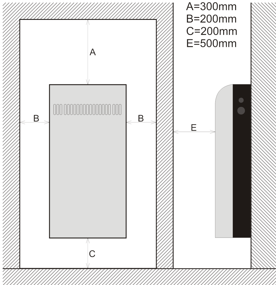
Slika: Minimalne udaljenosti prilikom montaže
