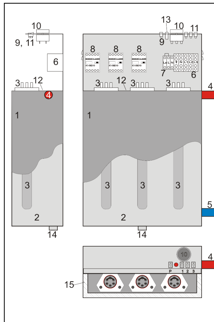
Slika: Sastavni delovi modela sa bočnim hidrauličnim priključcima
