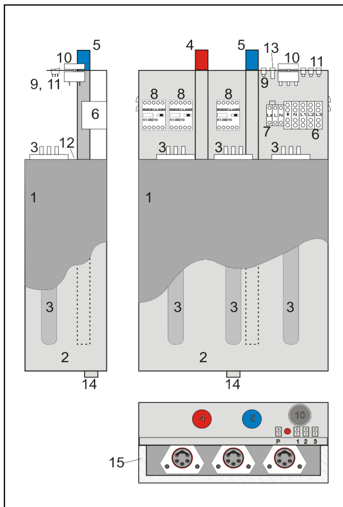
Slika: Sastavni delovi modela sa gornjim priključcima
