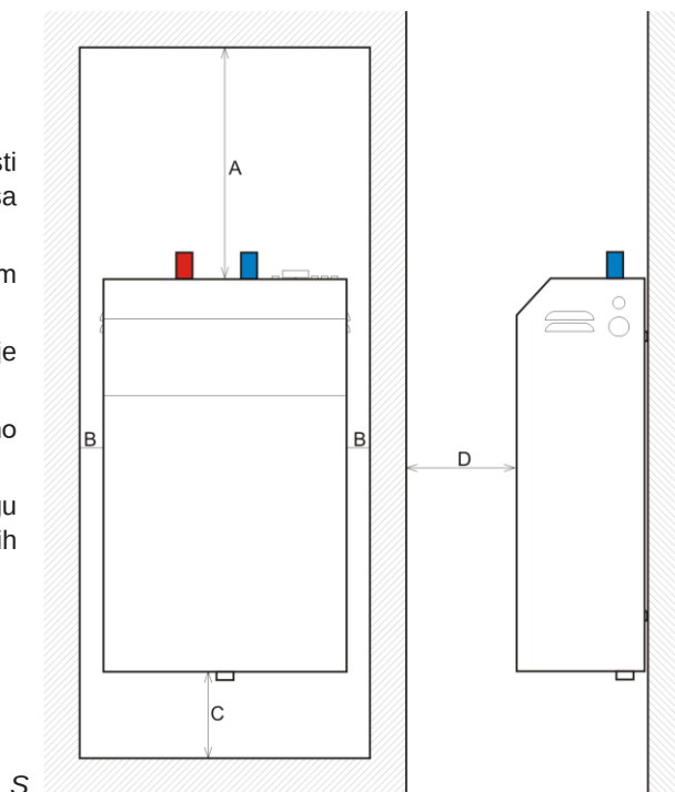
Slika 2 : Minimalna rastojanja prilikom montaže
