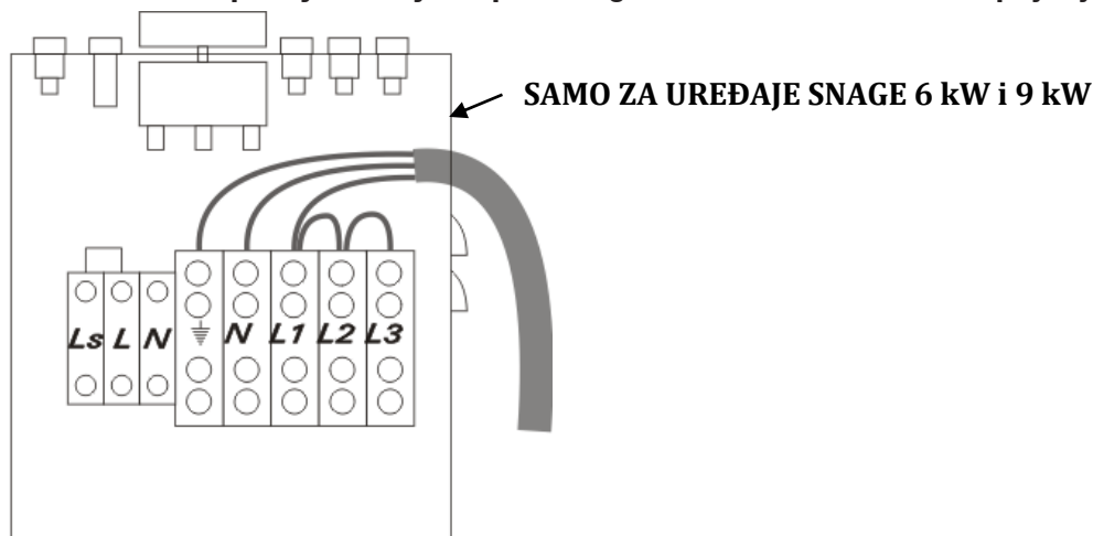
Slika 6: Shema priključivanja naponskog kabl na monofazno napajanje
