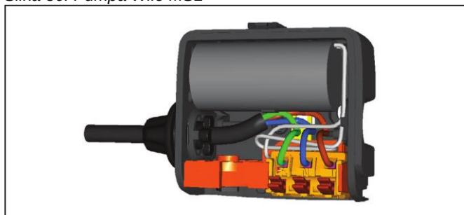
Slika 37: Povezivanje napojnog kabla pumpe
