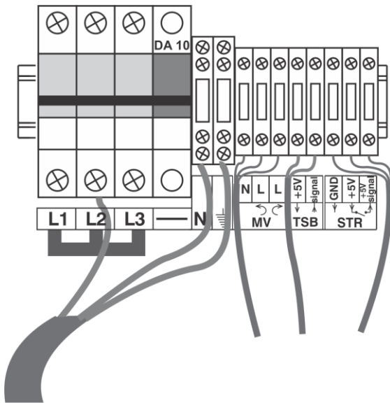
Montažna shema povezivanja kotla na monofazno električno napajanje SAMO ZA:
