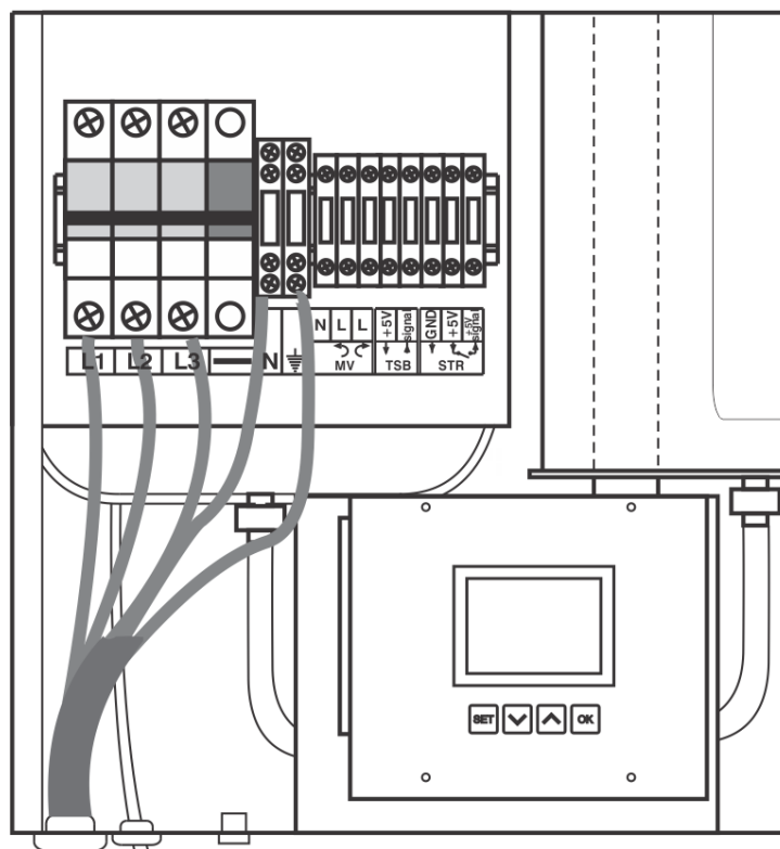
Slika 7: Shema spajanja električnih kablova
