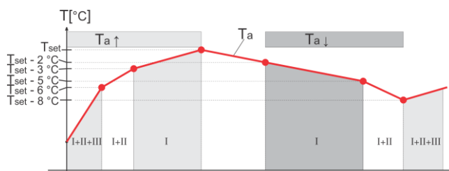
Slika 10: Uključivanje i isključivanje grejača
