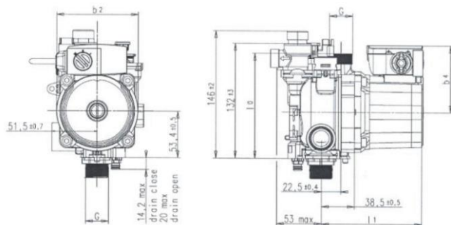
Slika 36: Pumpa Wilo MSL
