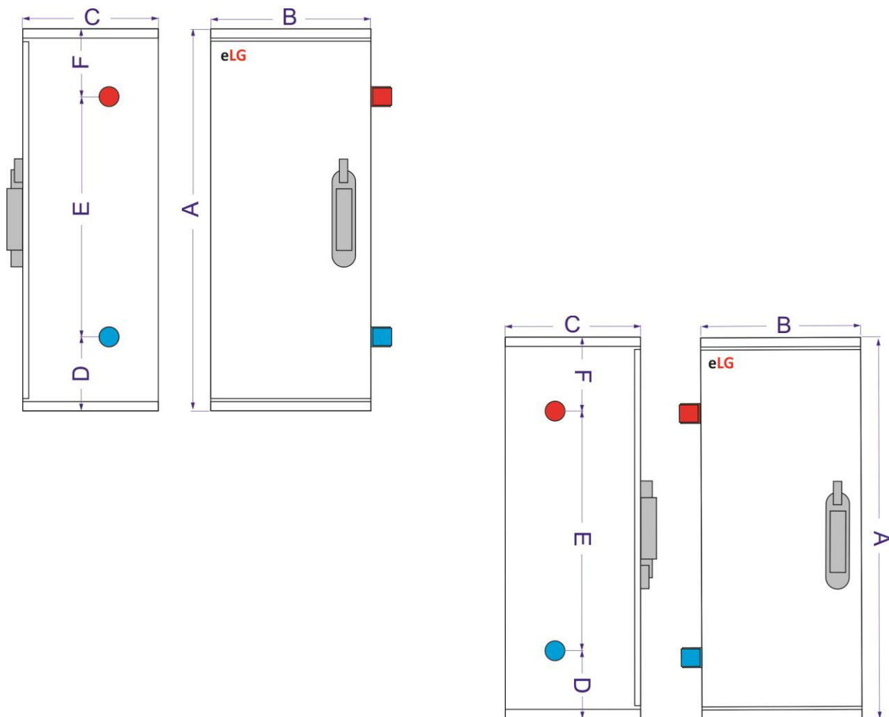
Slika Dimenzije kotla TK-eLG 6 kW – model IP54 za spoljašnju montažu sa hidrauličnim priključcima sa desne ili leve strane
