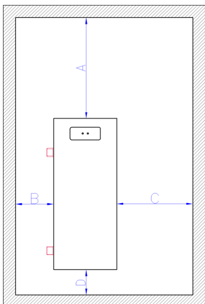
Slika 3a: Minimalne dimenzije slobodnog prostora za model sa hidrauličnim priključcima levo A = 500\text{mm} / B = 250\text{mm} / C = 500\text{mm} / D = 200\text{mm}
