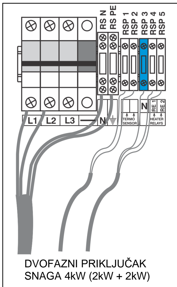
Slika6b Povezivanje na dve faze
