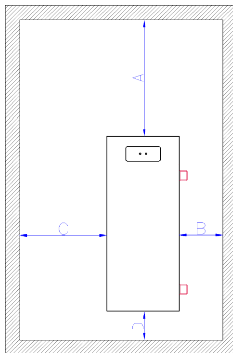
Slika 3b: Minimalne dimenzije slobodnog prostora za model sa hidrauličnim priključcima desno A = 500\text{mm} / B = 250\text{mm} / C = 500\text{mm} / D = 200\text{mm}
