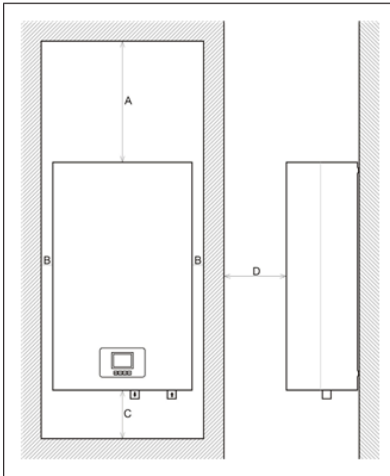
Slika/Image: Minimalne dimenzije slobodnog prostora za montažu/ Minimum dimensions of free mounting space: A = 500mm / B = 50mm / C = 200mm / D = 500mm
