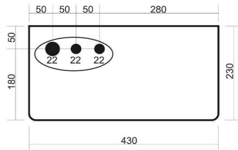
Slika/Image: Prikaz pozicija uvodnika kablova na kotlu mTronic7000 / Display of cable gland positions on the mTronic7000 boiler
