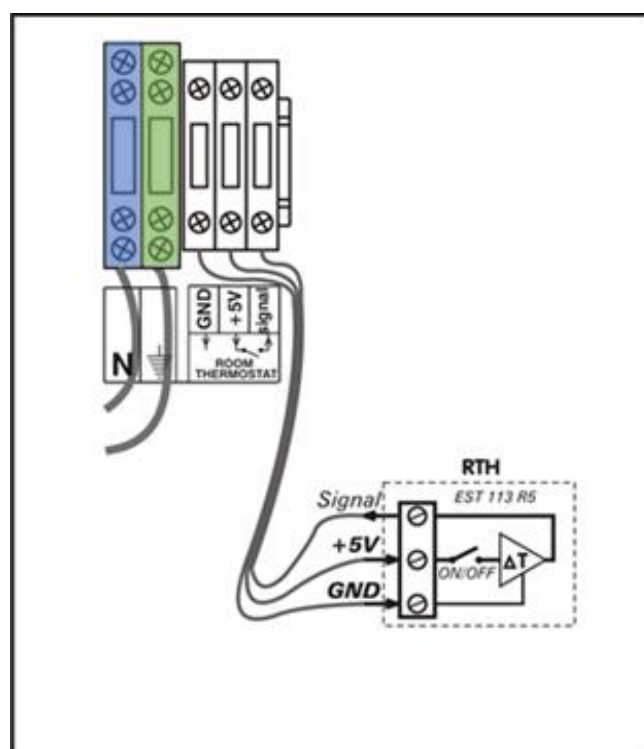
11. ábra: Az EST 113 R5 szobatermosztát csatlakoztatási vázlata
