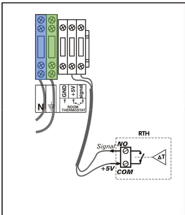
10. ábra: Digitális programozású elemes tápellátású szoba termosztát csatlakoztatási vázlata
