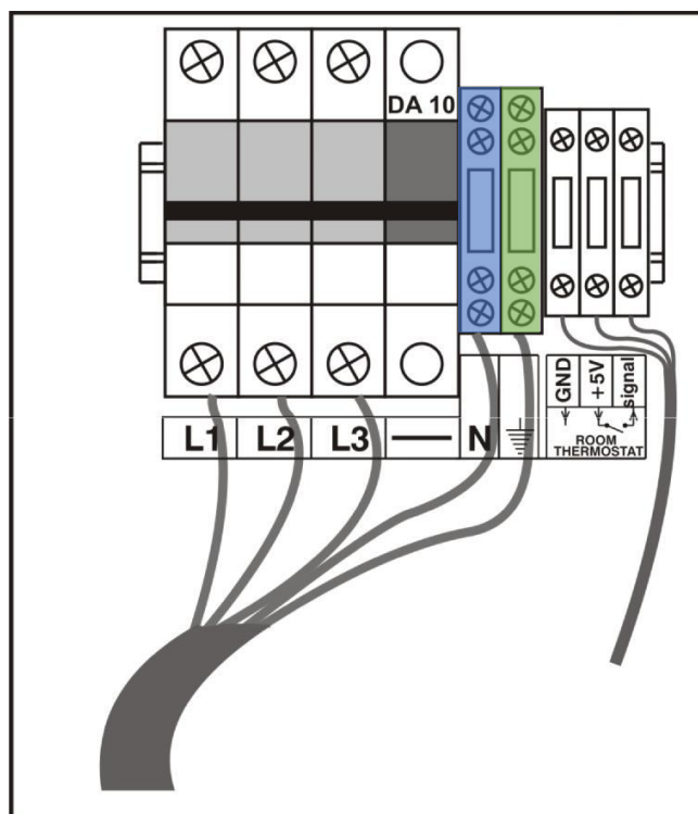
Imaginea 9: Siguranțe ETI
