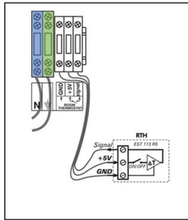
Imaginea 11: Schema de conectare la termostat de cameră MIKOTERM EST 113 R5
