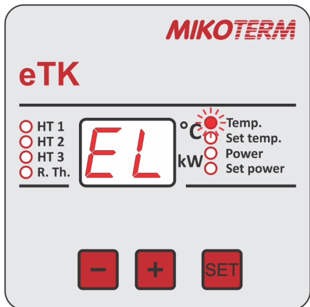
Imaginea23: Temperatura sub -9^{\circ}\text{C} sau scurt circuitul de senzor
