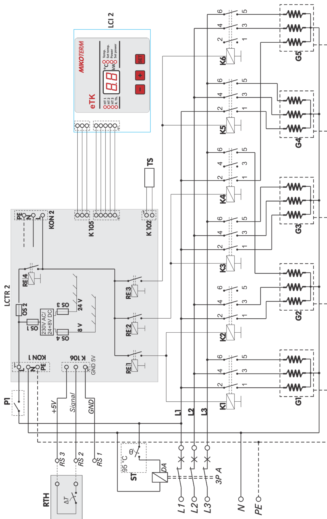
Imaginea 14: Schema electrică a centralei eTK de puterea nominală 30kW, 36kW and 40kW
