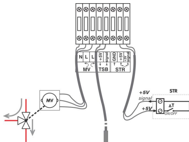
Шема за спојување на термостатот на загреаната просторија, сонда за мерење на температура во резервоарот и моторниот 3-патен вентил (230V 50Hz).
