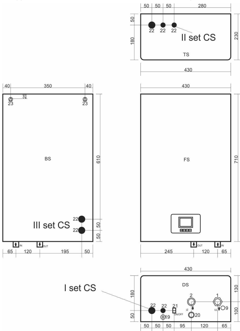
I set CS / II set CS / III set CS – Позиција на првиот сет на држачи за кабел
