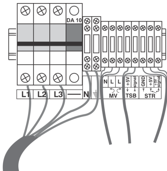
Slika 9: Povezivanje električnog napajanja kod ETI osigurača Montažna shema povezivanja kotla na trofazno električno napajanje
