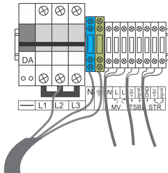
Bild 9b: NOARK-Sicherungen
