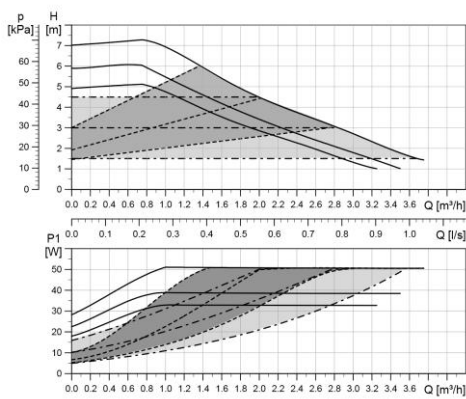
Kennlinie der Pumpe Grundfos UPM3 AUTO
