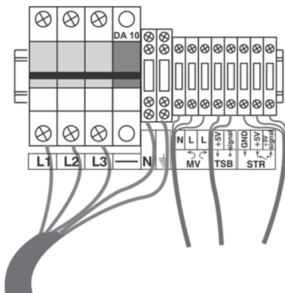
Bild 9a: ETI-Sicherungen
