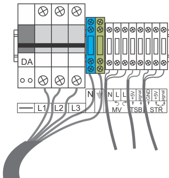
Bild 9c: NOARK-Sicherungen
