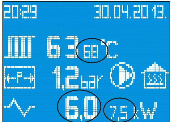
Bild 14: Einstellung der Betriebstemperatur des Kessels
